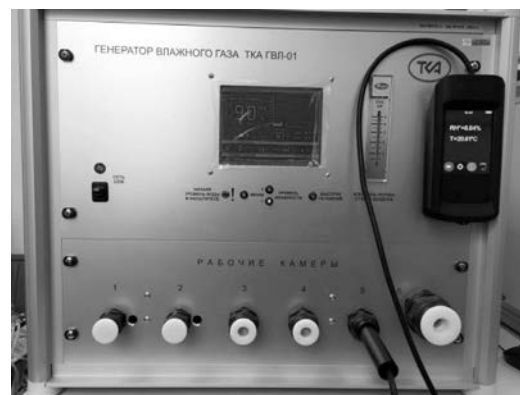
Рис. 5. Термогигрометр эталонный ТКА-ТВ/Эталон в составе генератора влажности ТКА-ГВЛ-01
